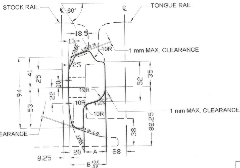
END ELEVATION XX
