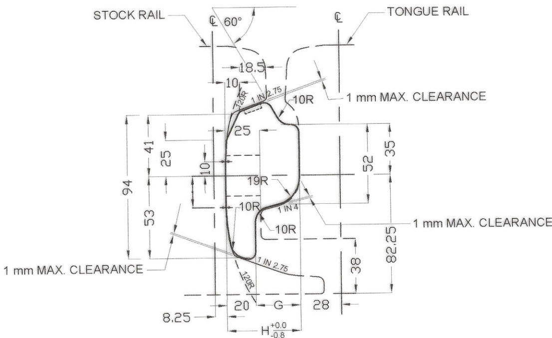
END ELEVATION Y'Y'
