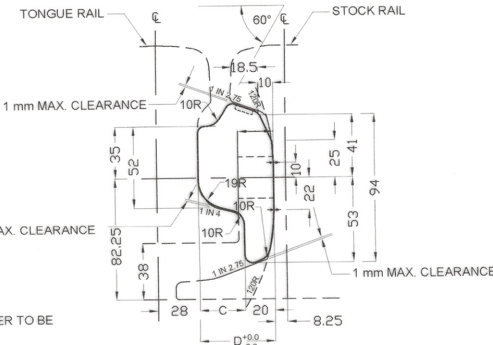
END ELEVATION YY
